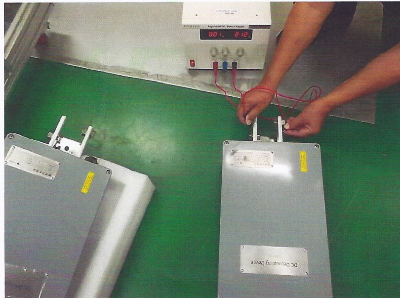
Photo. SG02 : 서지전류시험
